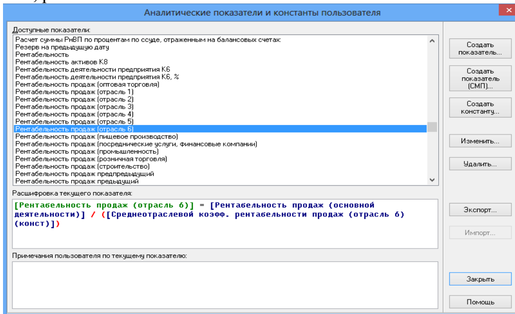
Рис. 29. Аналитические показатели и константы пользователя
