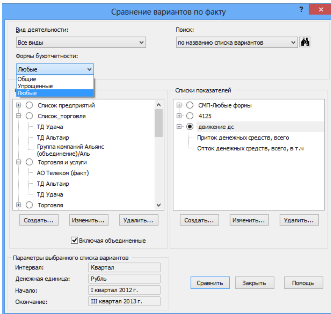
Рис. 33. Сравнение вариантов по факту
